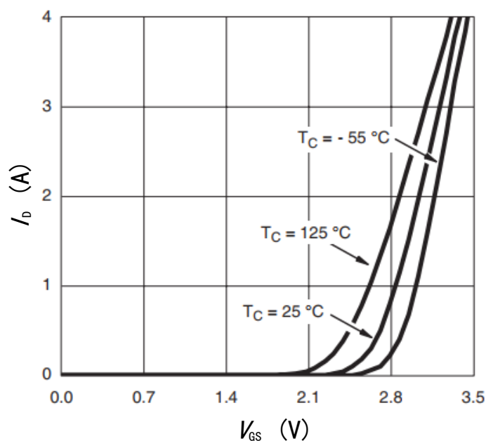
图 2 转移特性曲线
