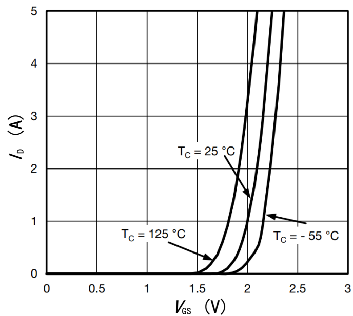
图 2 转移特性曲线
