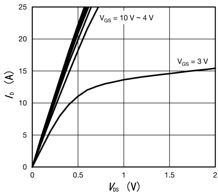
图 1 开启区域特性曲线
