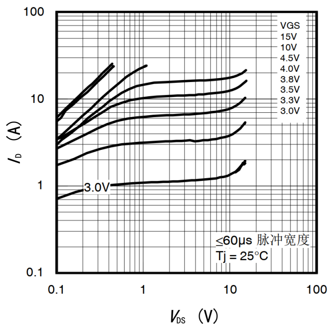
图 1 开启区域特性曲线
