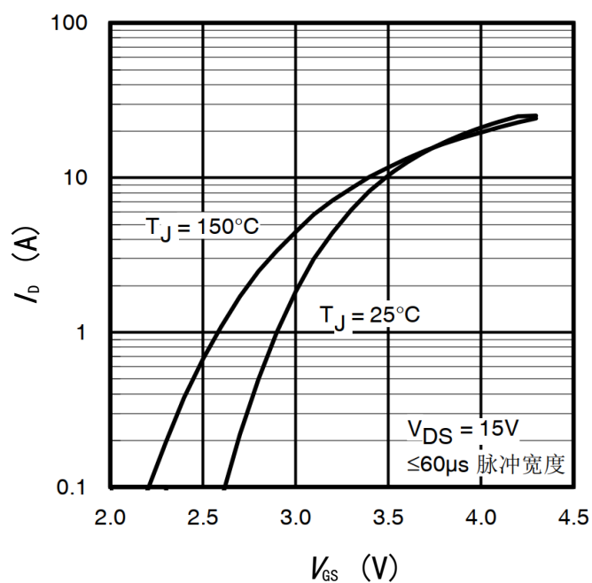
图 2 转移特性曲线
