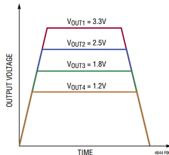
图 3 输出重合跟踪波形
