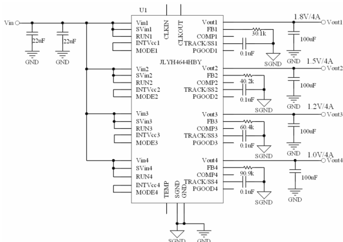
图 4 输入 12V，四路（1.8V/4A、1.5V/4A、1.2V/4A、1.0V/4A）输出
