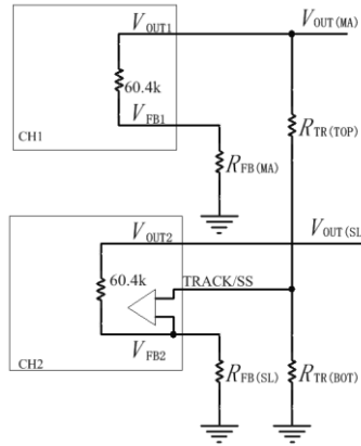
图 2 输出电压跟随示意图
