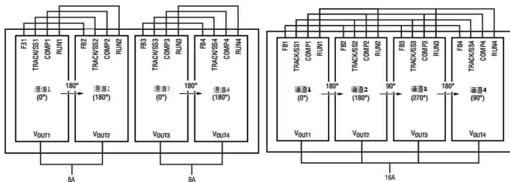
图 5 2+2 和 4 通道并联示意图
