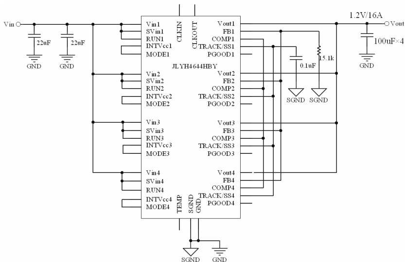
图 6 输入 4V~14V，四路并联（1.2V/16A）输出
