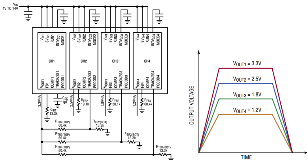
图 1 输出比例式跟踪原理图和输出波形
