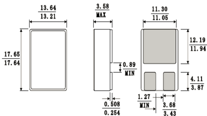
图 6 SMD-2 外形尺寸
