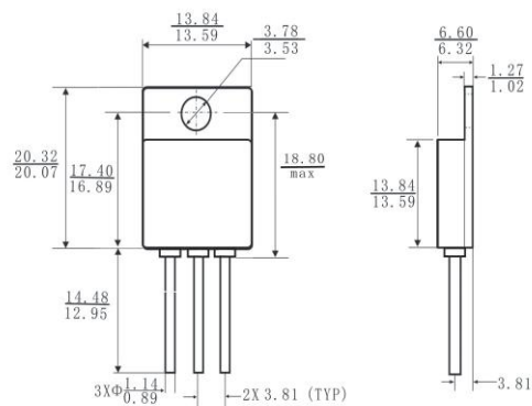
图 4 T0-254 外形尺寸
