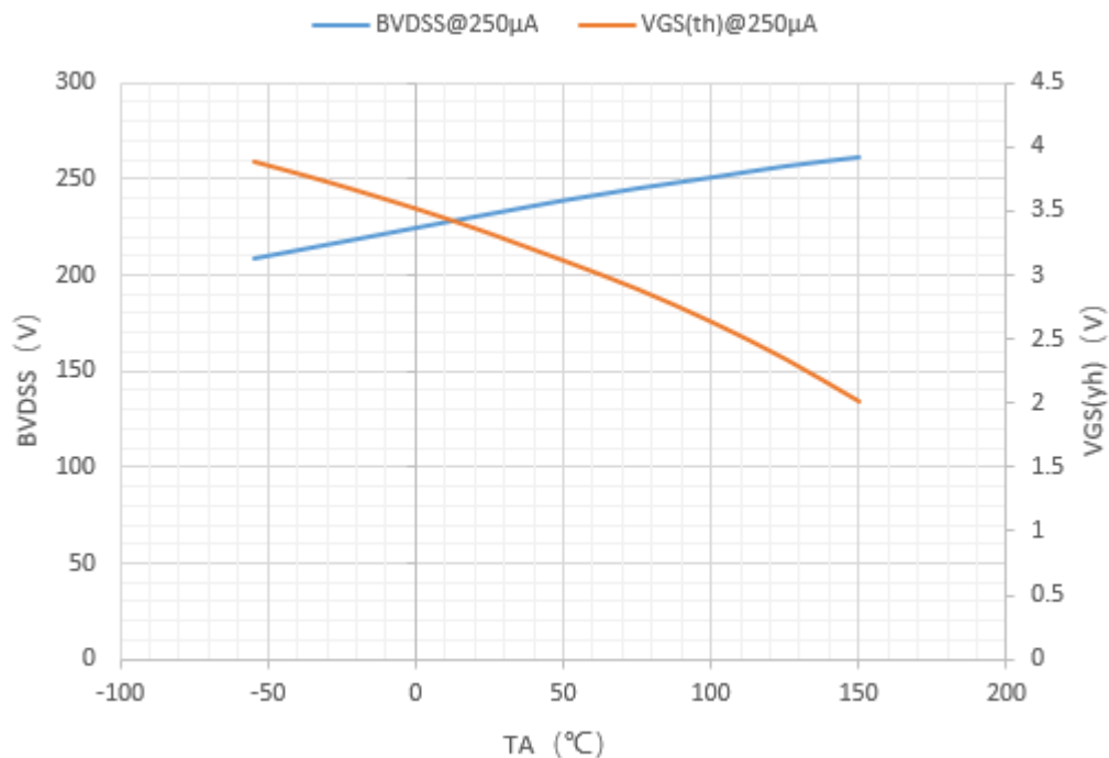
图 2 漏源击穿电压、阈值电压特性曲线
