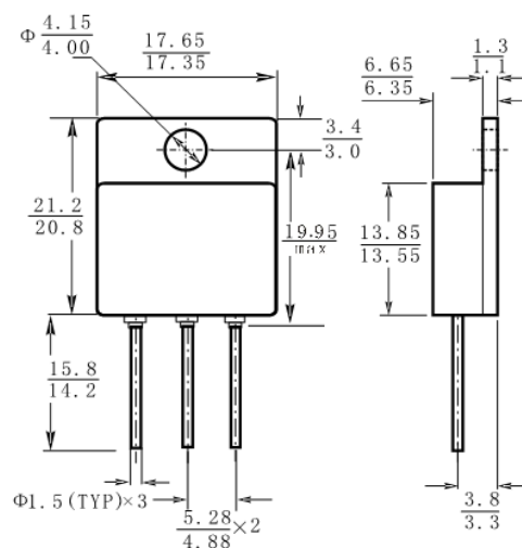
图 5 T0-258 外形尺寸
