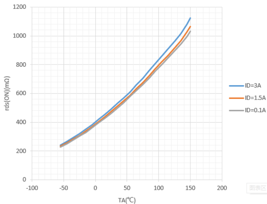
图 1 导通电阻特性曲线
