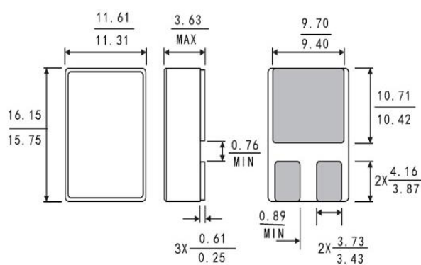
图 6 SMD-1 外形尺寸
