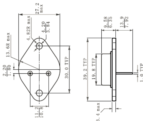
图 7 B2-01C 外形尺寸
