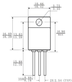
图 4 T0-257 外形尺寸
