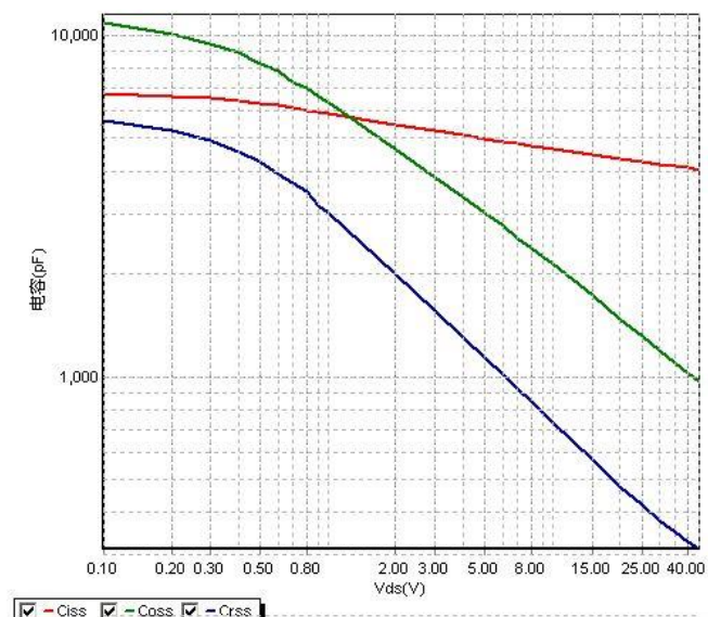
图 4 电容特性曲线
