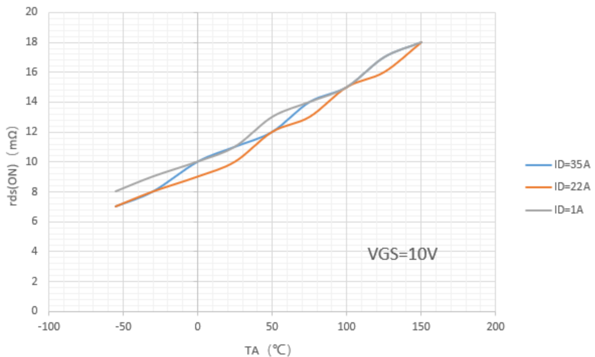
图 1 导通电阻特性曲线
