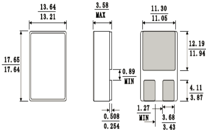
SMD-2 外形尺寸
