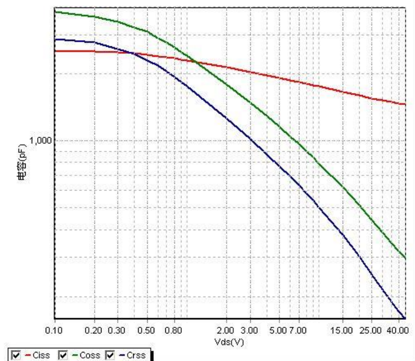
图 4 电容特性曲线
