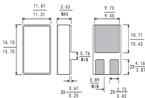
图 7 SMD-1 外形尺寸
