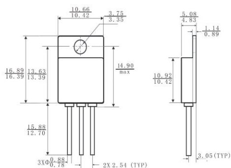
图 5 T0-257 外形尺寸
