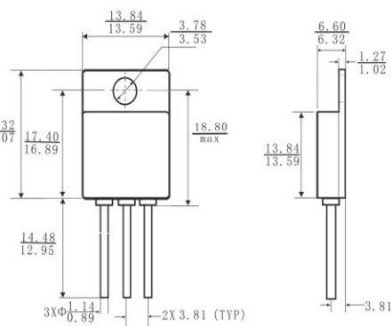
图 6 T0-254 外形尺寸
