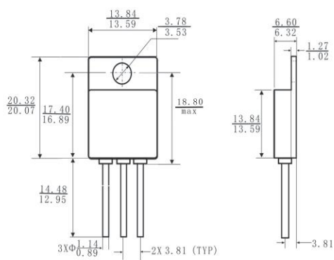
图 5 T0-254 外形尺寸
