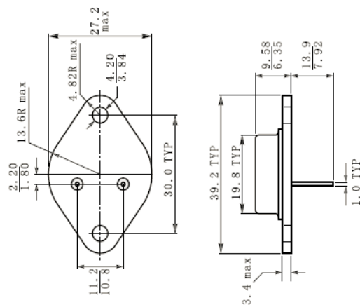
图 6 B2-01C 外形尺寸
