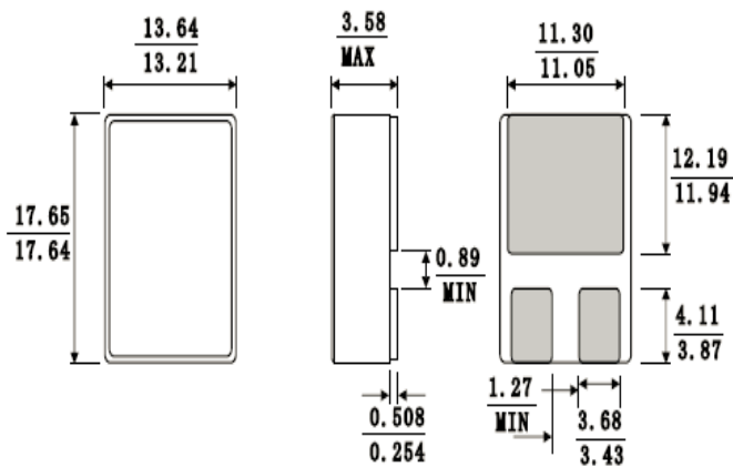
图 7 SMD-2 外形尺寸
