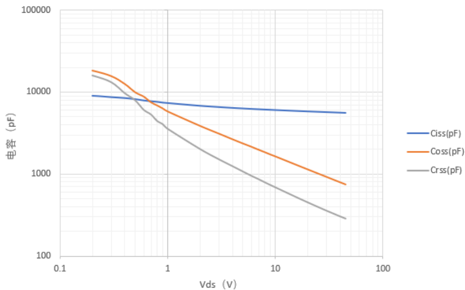
图 4 电容特性曲线
