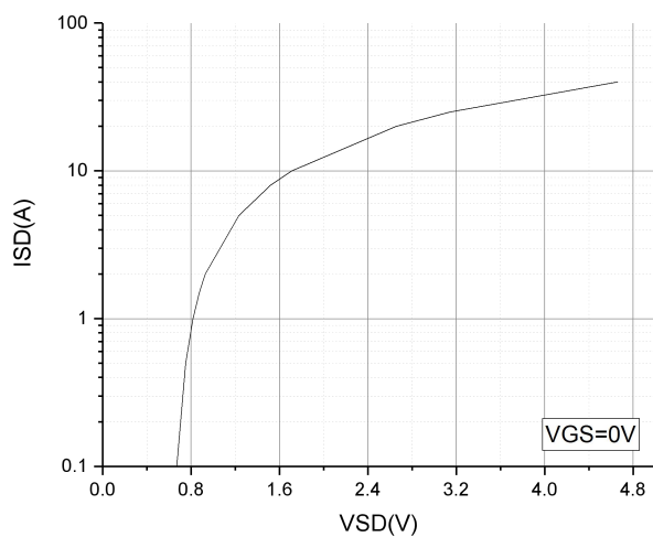
图 5 体二极管特性曲线
