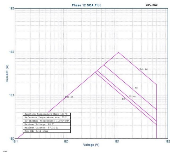
图 6 安全工作区曲线
