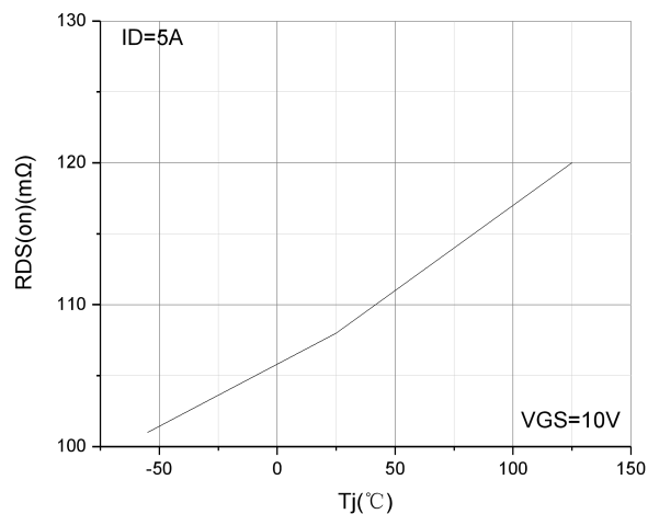
图 2 R_{DS(on)} - T_J 曲线
