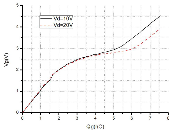
图 4 V_{GS} - Q_g 特性曲线
