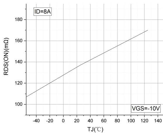
图 2 R_{DS(on)} - T_J 曲线
