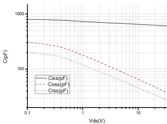
图 3 C - V_{DS} 特性曲线
