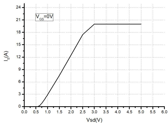
图 2 体二极管特性曲线
