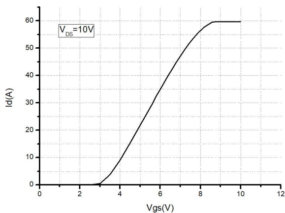
图 1 转移特性曲线
