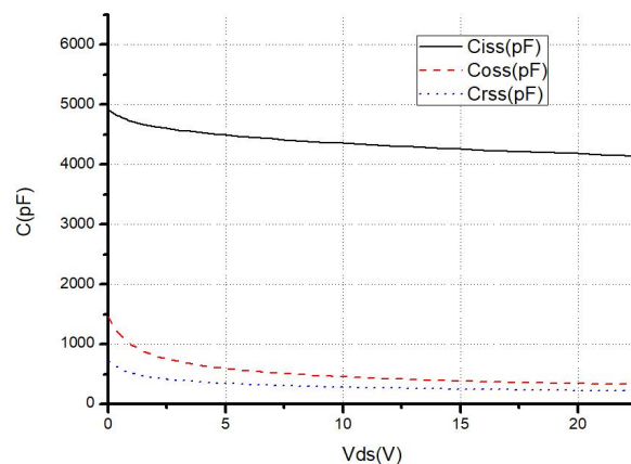
图 4 C-V_{DS} 特性曲线
