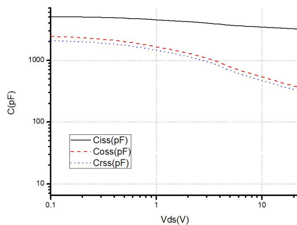
图 4 C-VDS 特性曲线
