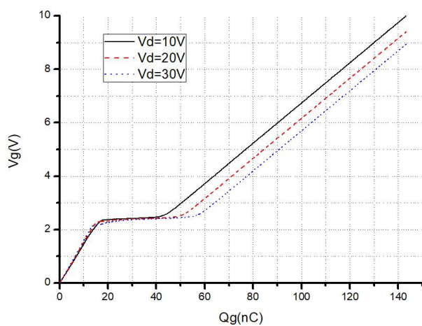
图 3 VGS-Qg 特性曲线
