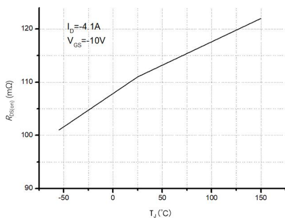
图 5 R_{ds(on)}-T_j 特性曲线
