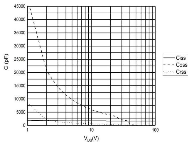
图 4 电容曲线
