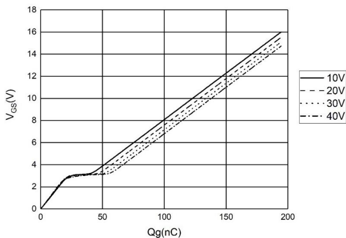
图 5 V_{GS}-Q_g 特性曲线
