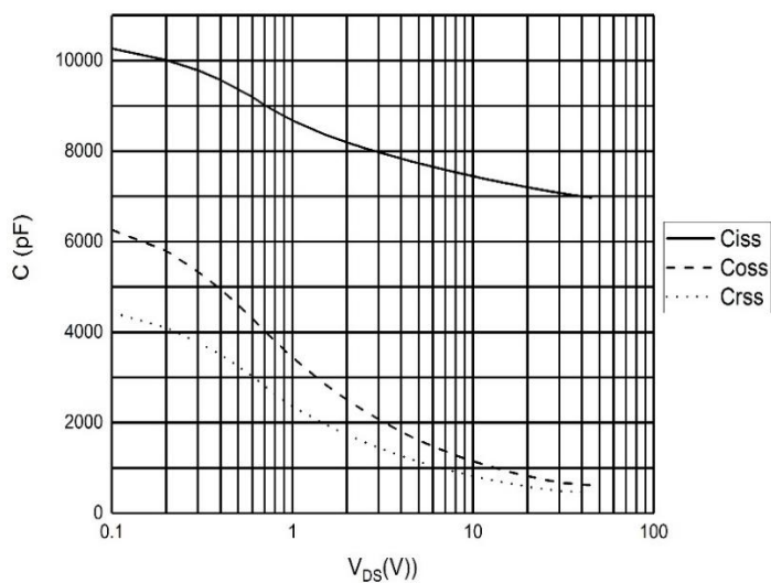
图 4 电容曲线
