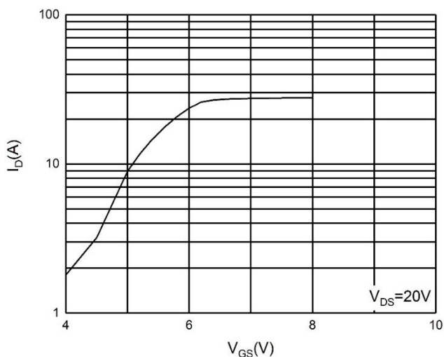
图 1 转移特性曲线
