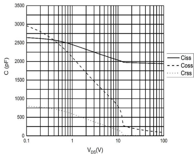
图 4 电容曲线
