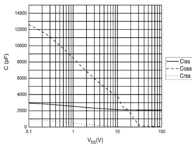
图 4 电容曲线
