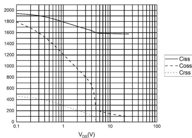
图 4 电容曲线
