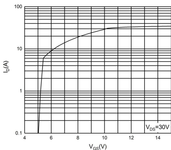
图 1 转移特性曲线
