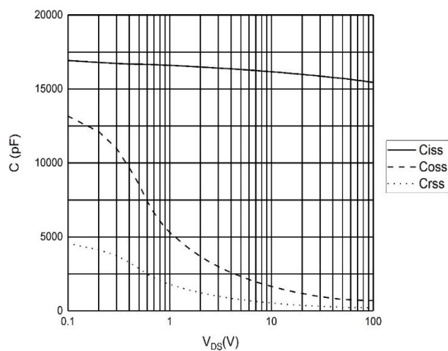
图 4 电容曲线
