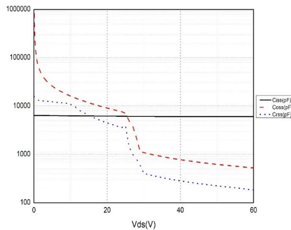
图 4 电容曲线
