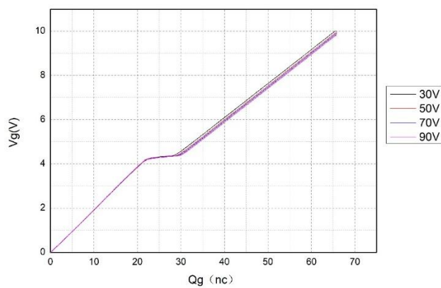
图 5 特性曲线
