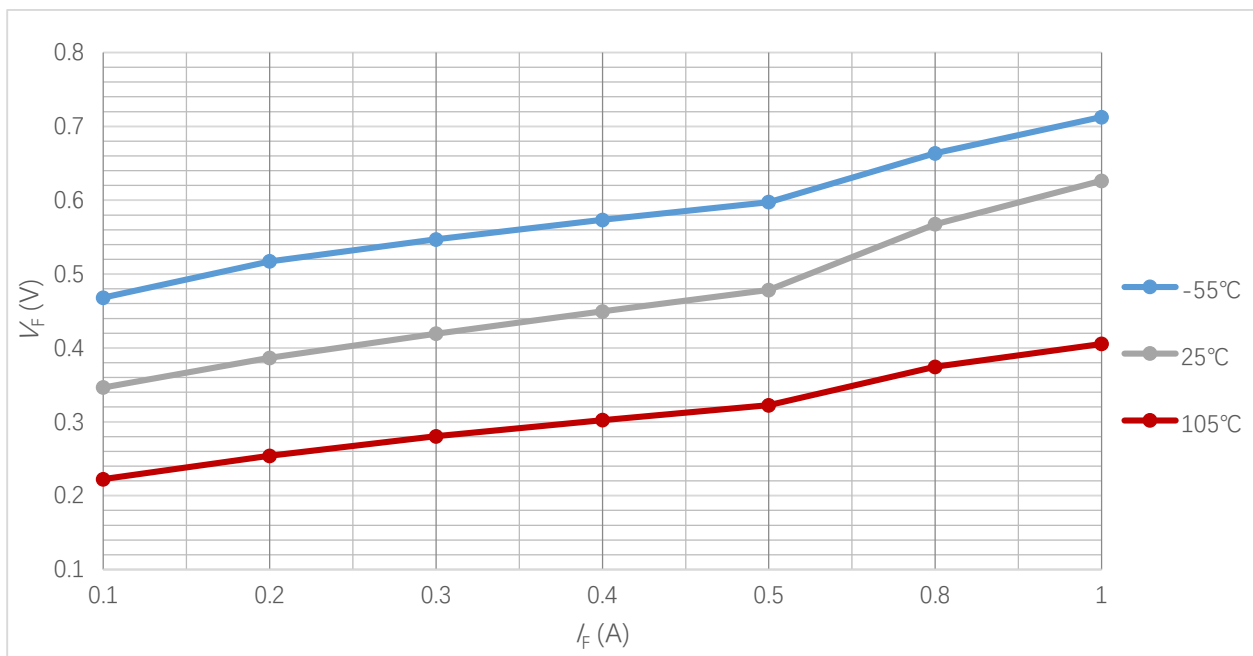
图2 V_F — I_F 特性曲线
