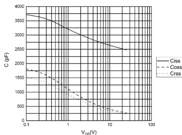
图 4 电容曲线
