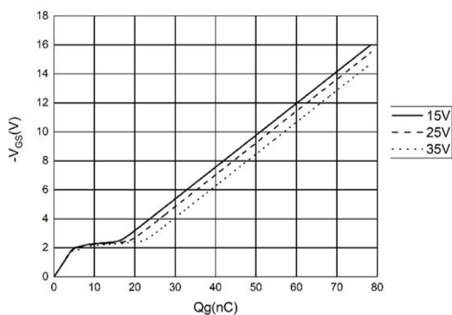
图 5 特性曲线
