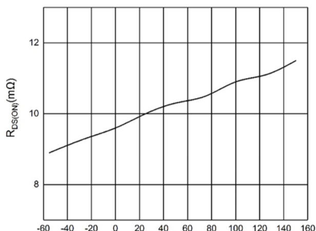
图 3 R_{DS(on)}-T_J 特性曲线
