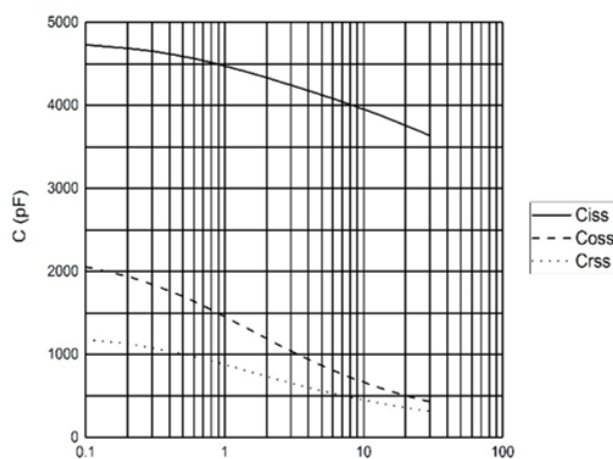
图 4 电容曲线
