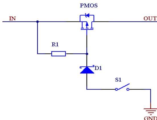
图 9 典型开关电路
