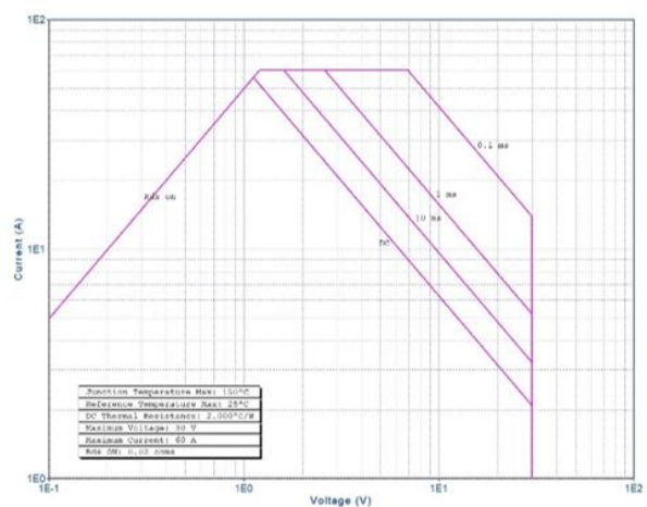
图 6 安全工作区曲线
