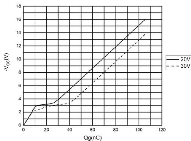
图 5 特性曲线
