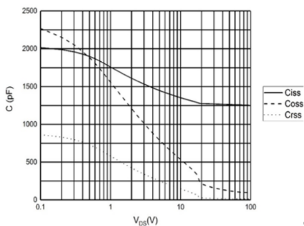
图 4 电容曲线
