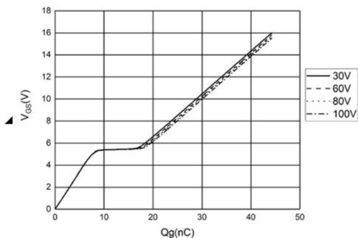
图 5 特性曲线
