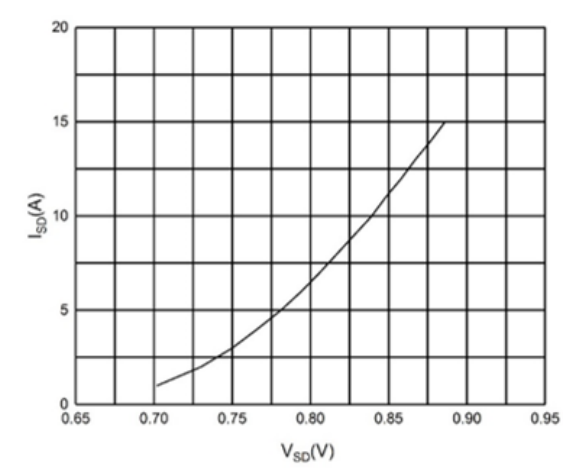
图 2 体二极管特性曲线
