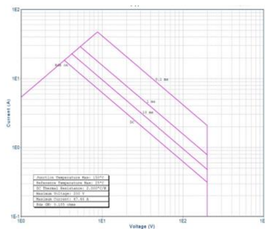
图 6 安全工作区曲线
