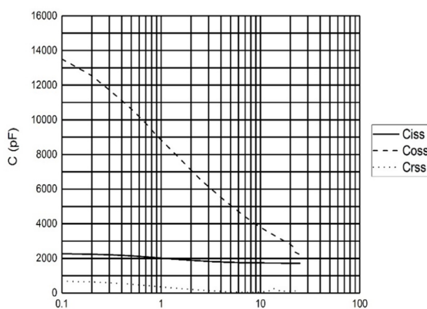
图 4 电容曲线
