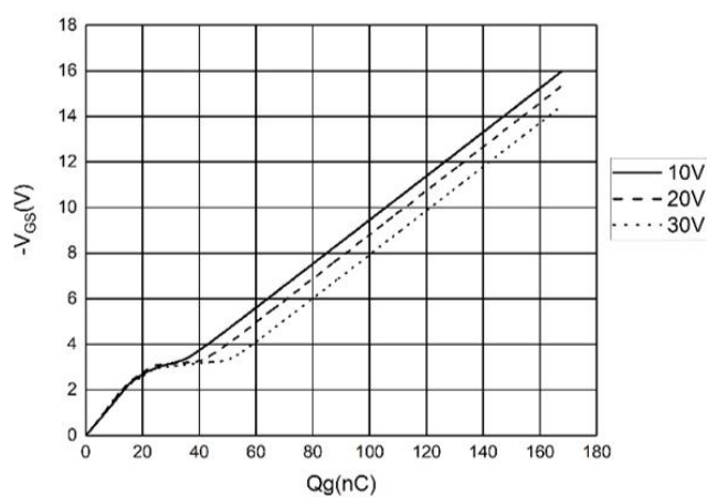
图 5 特性曲线
