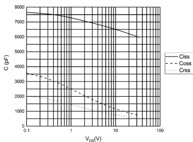
图 4 电容曲线
