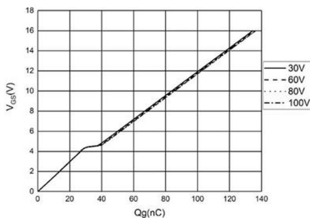
图 5 特性曲线
