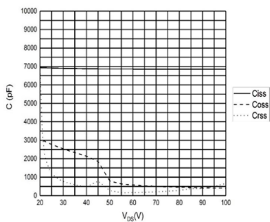
图 4 电容曲线
