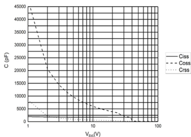
图 4 电容曲线
