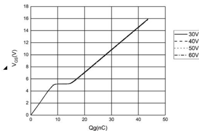
图 5 特性曲线
