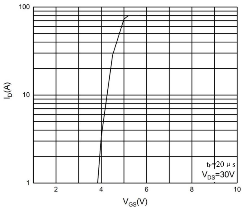
图 1 转移特性曲线
