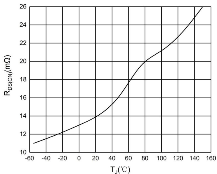
图 3 R_{DS(on)}-T_J 特性曲线
