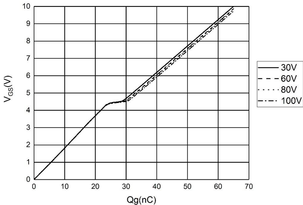
图 5 V_{GS}-Q_g 特性曲线
