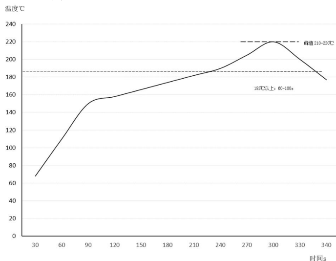
图 11 建议的回流焊曲线
