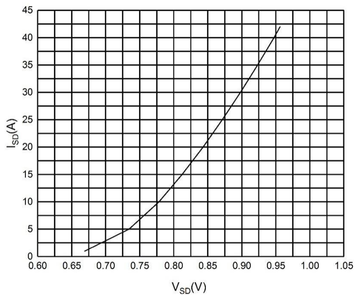
图 2 体二极管特性曲线
