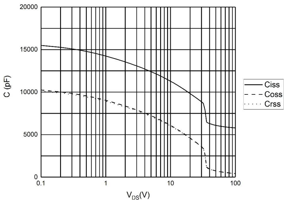
图 4 电容曲线
