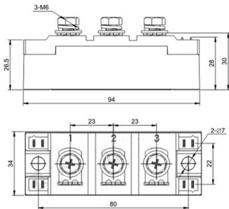
图 1 D0012A 外形尺寸图
