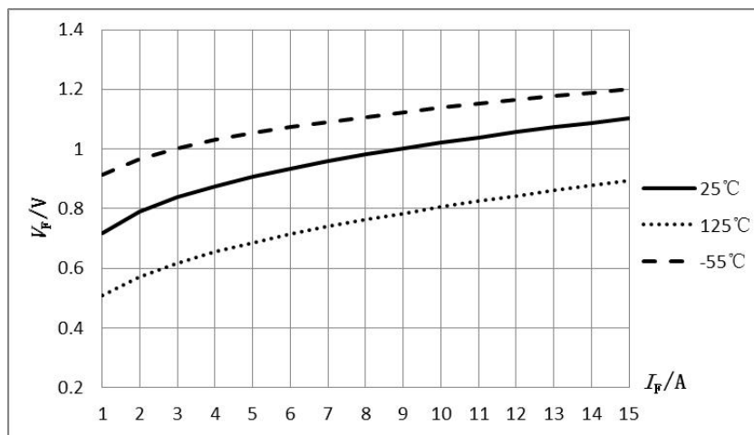
图 2 I_F-V_F 特性曲线
