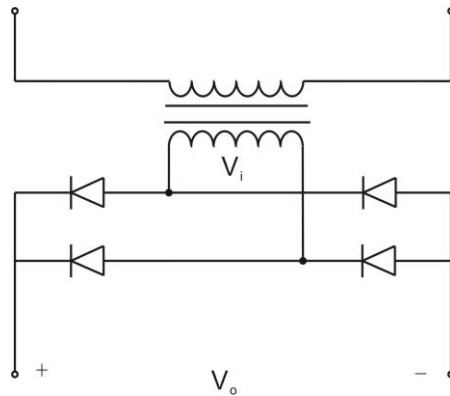
图 7 单相全波整流电路
