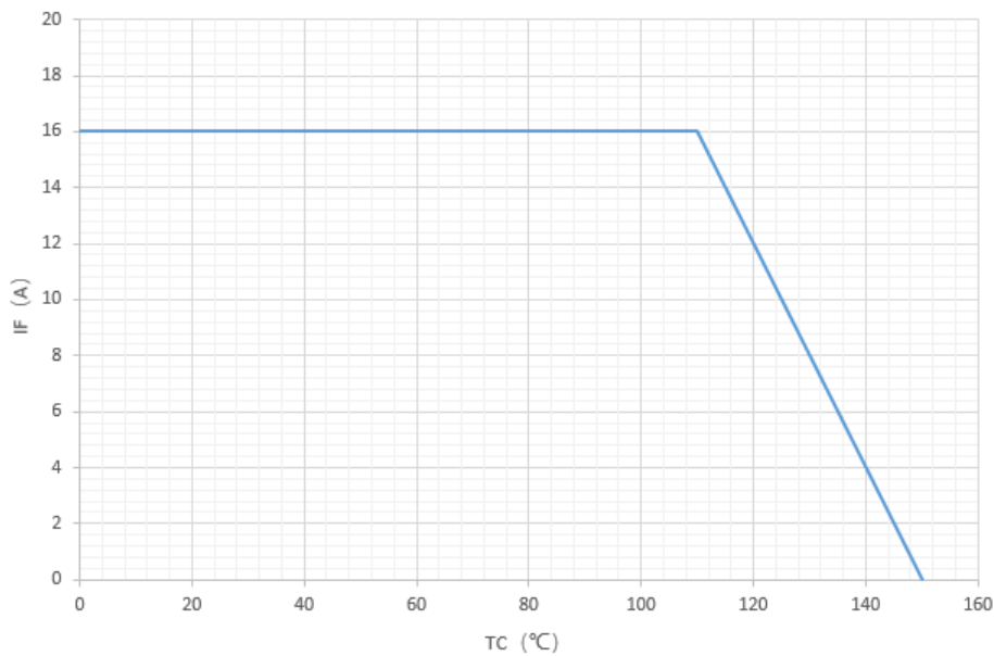
图 4 正向电流降额曲线
