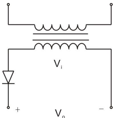
图 6 单相半波整流电路
