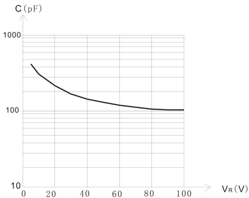
图3 C_{tot} — V_R 特性曲线
