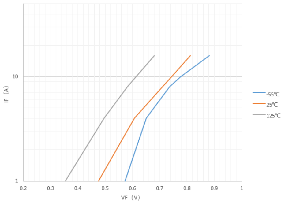
图2 V_F — I_F 特性曲线
