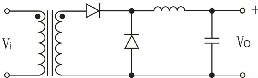
图 8 整流加续流电路
