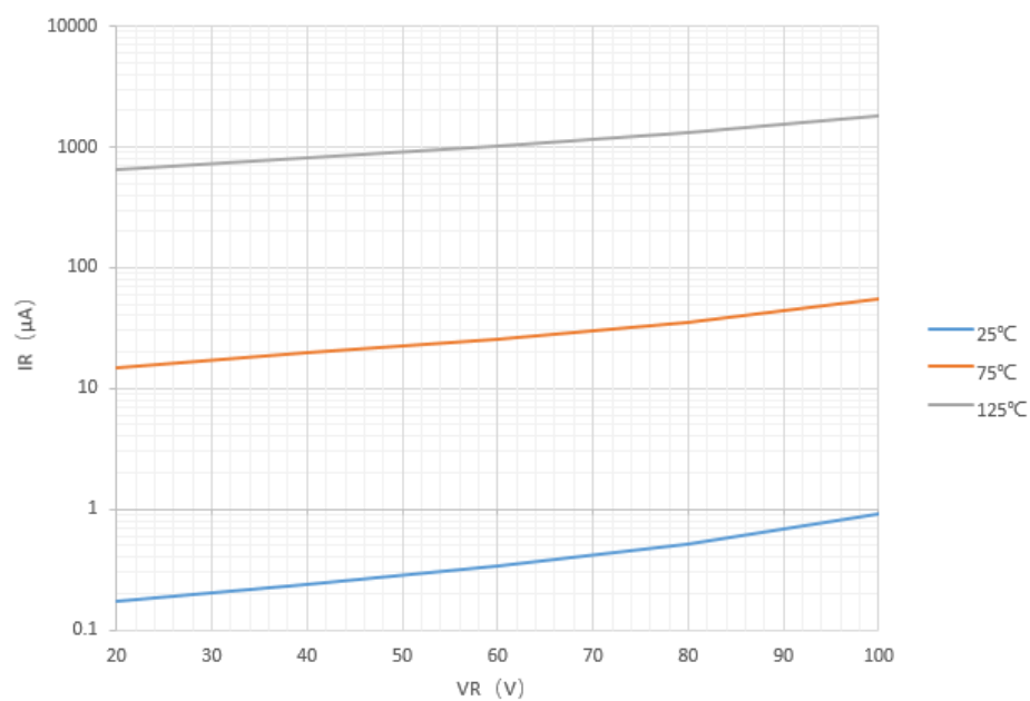
图 1 I_R-V_R 特性曲线
