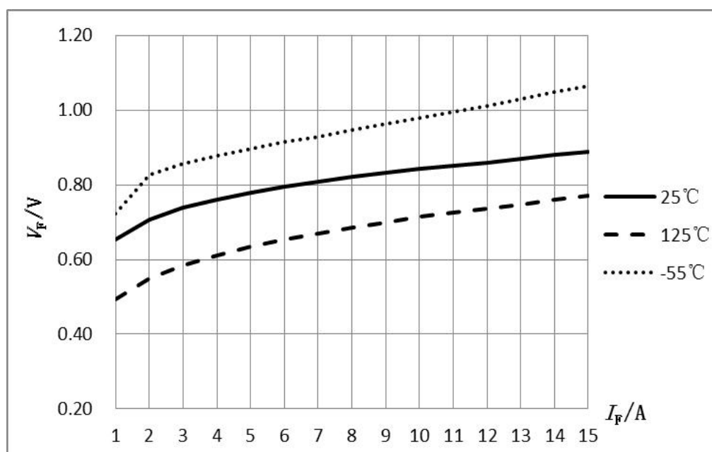
图2 V_F-I_F 特性曲线
