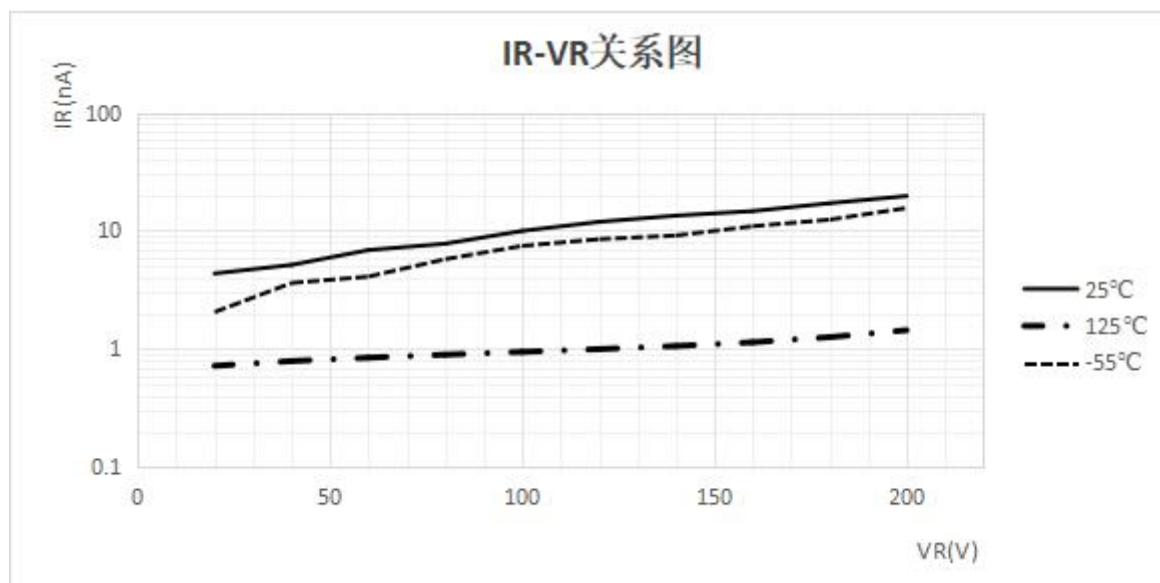
图1 I_R-V_R 特性曲线
