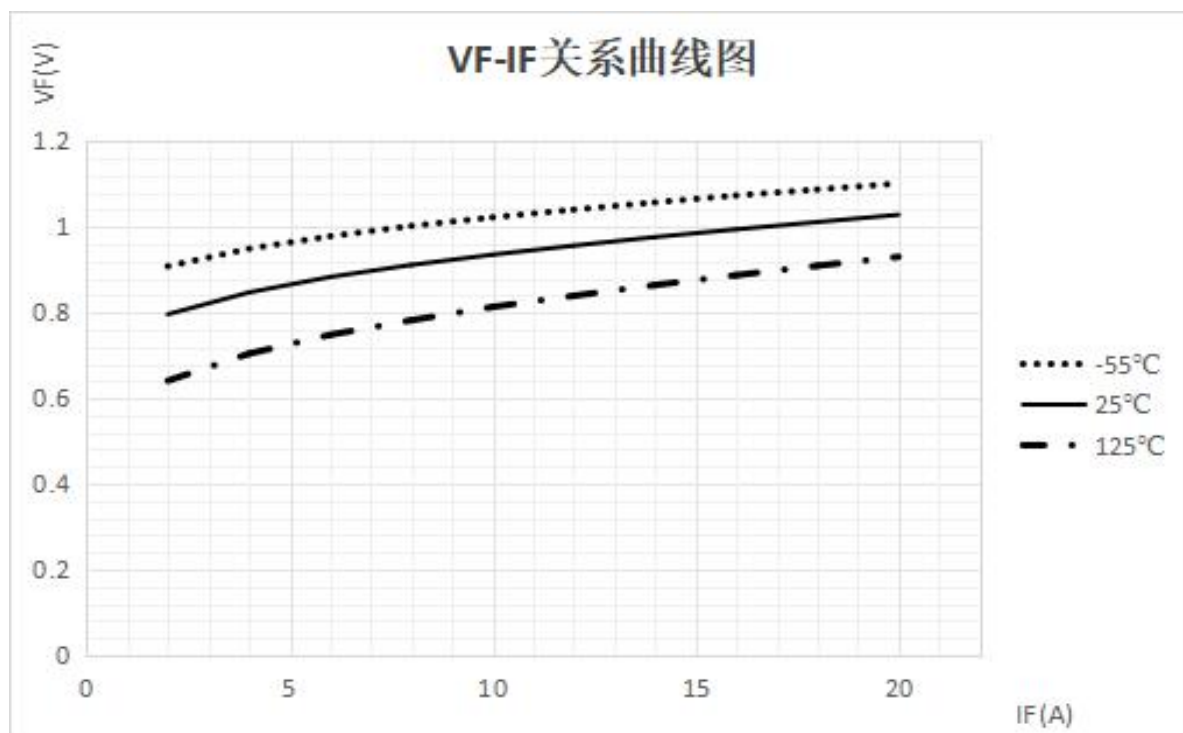
图2 V_F-I_F 特性曲线
