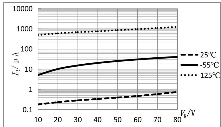
图1 I_R - V_R 特性曲线
