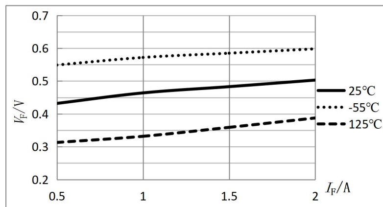
图2 V_F - I_F 特性曲线
