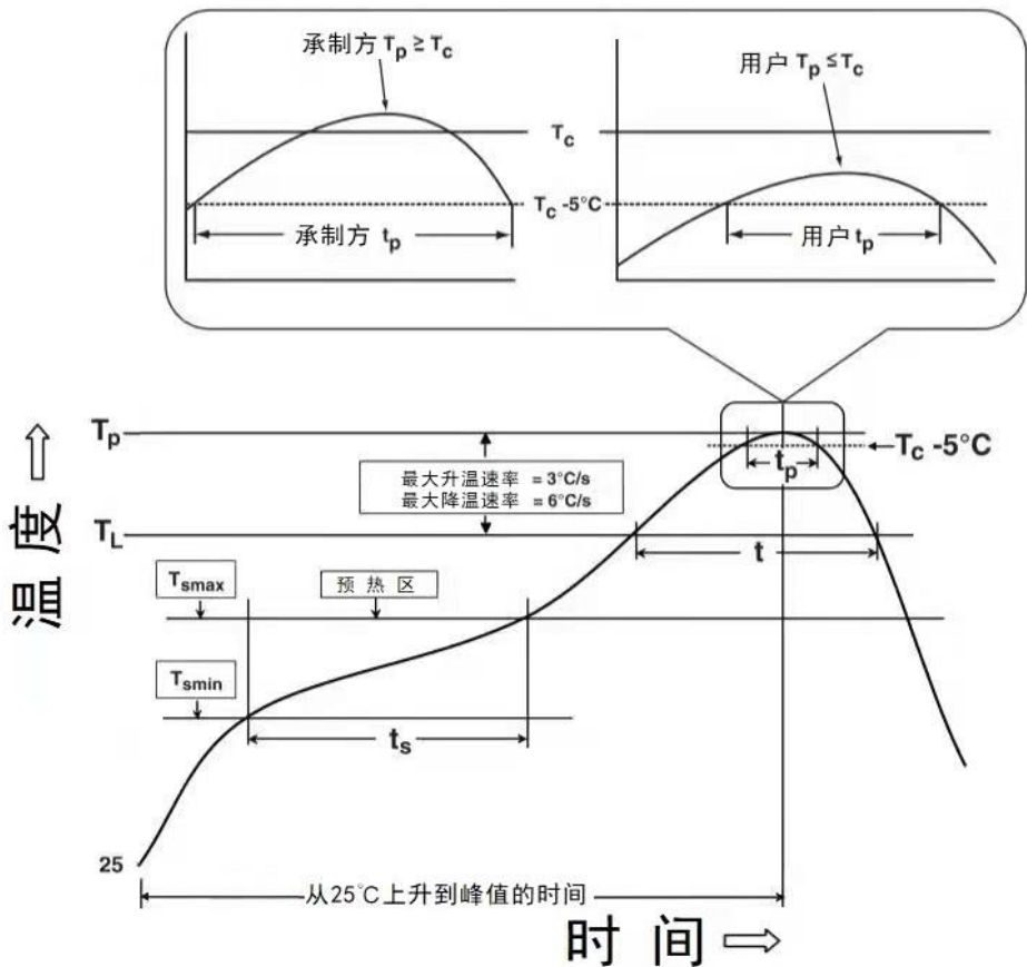
图 8 回流温度-时间分布图
