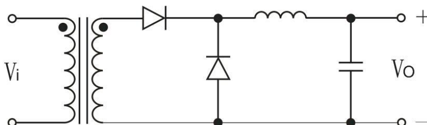
图 7 整流加续流电路
