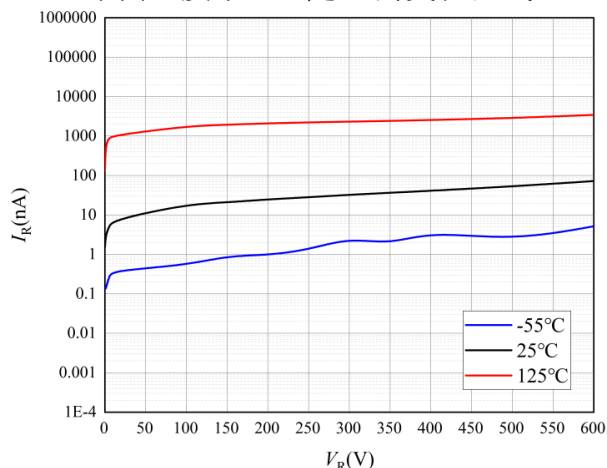
图 2 反向特性曲线
