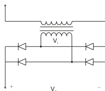
图 6 单相全波整流电路
