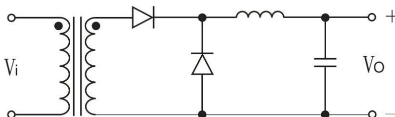
图 7 整流加续流电路
