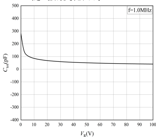
图 3 结电容特性曲线
