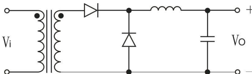
图 7 整流加续流电路
