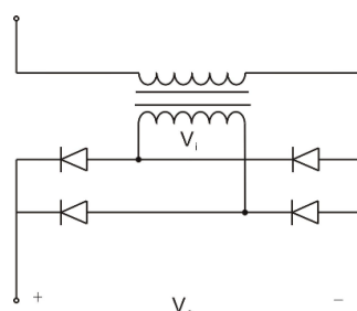
图 6 单相全波整流电路
