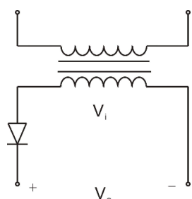
图 5 单相半波整流电路图
