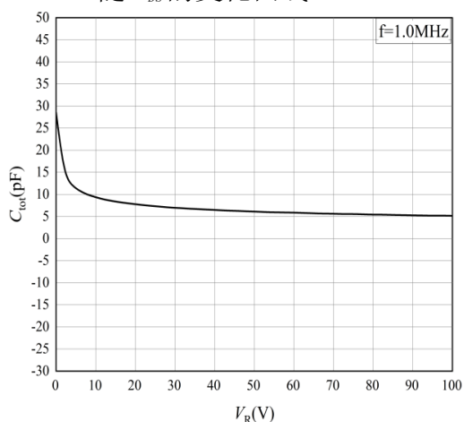
图 3 结电容特性曲线
