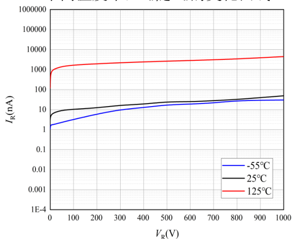
图 2 反向特性曲线
