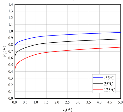
图 1 正向特性曲线
