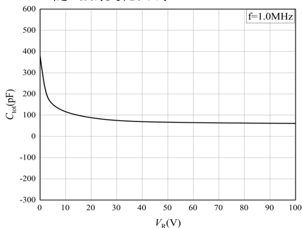
图 3 结电容特性曲线
