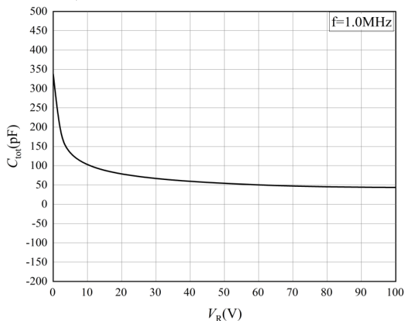
图 3 结电容特性曲线
